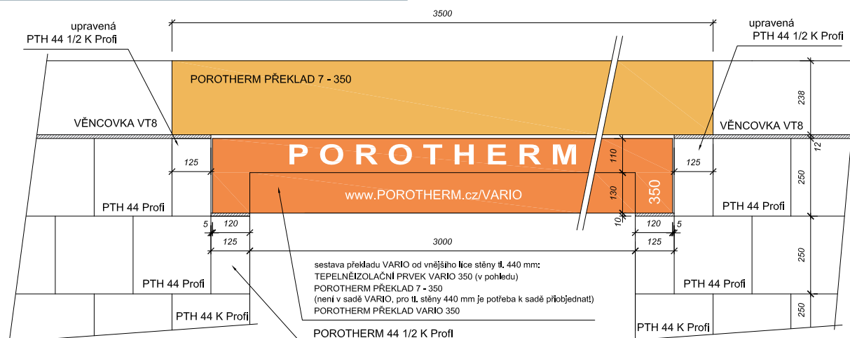
Sestava překladů pro světlost otvoru 3000 mm - pohled zvenku
