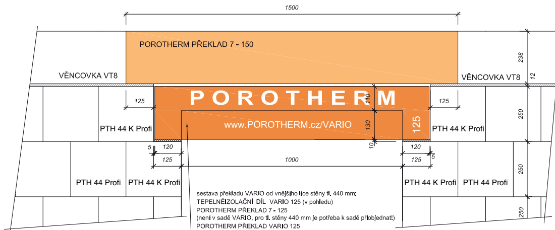
Sestava překladů pro světlost otvoru 1000 mm - pohled zvenku
