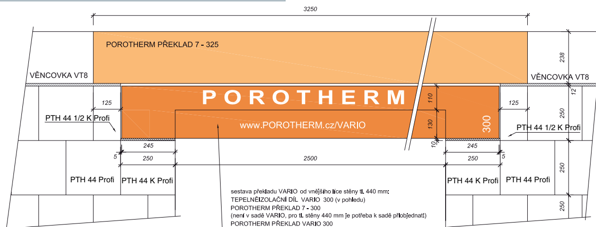
Sestava překladů pro světlost otvoru 2500 mm - pohled zvenku
